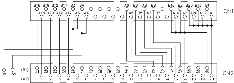
Wiring Diagram:
